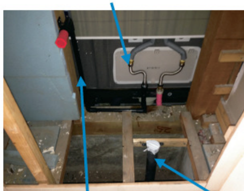
手洗い水栓給水管
