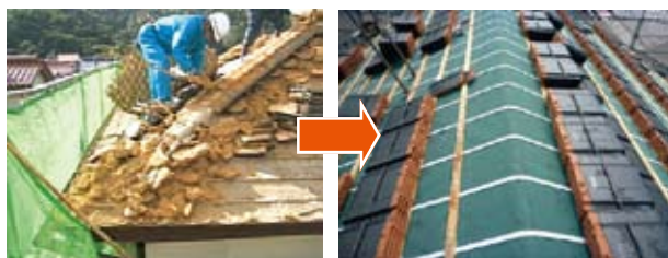
土葺き屋根 ⇒ 桟掛け瓦葺き
